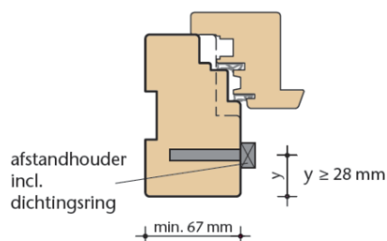
Bevestigingspunt B (in de dag van het kozijn)
